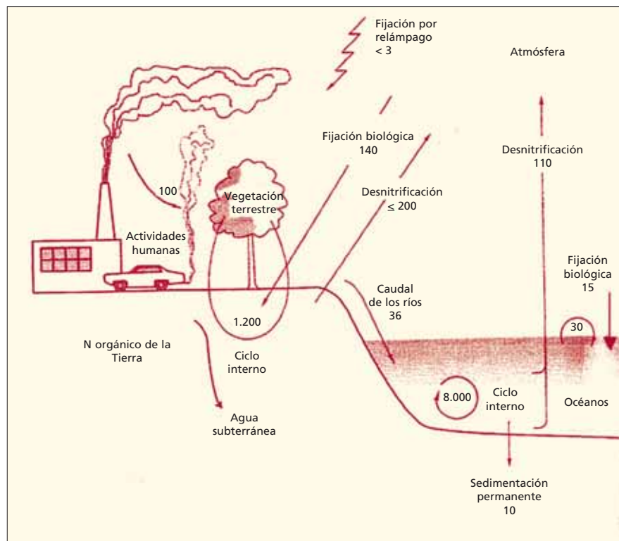
Figura 4.5. El ciclo global del nitrógeno, mostrando la conexión entre atmósfera, tierra y océano. Los flujos (representados por flechas) están en Tg ( 10^{12} g) N año ^{-1} y los reservorios representados por cajas en Tg N.
